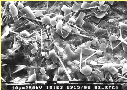
Magnification 1 : 1010
